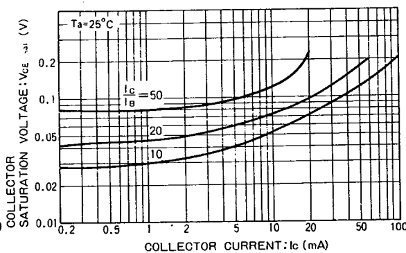
Fig.6 コレクタ・エミッタ飽和電圧-コレクタ電流特性 (I)
