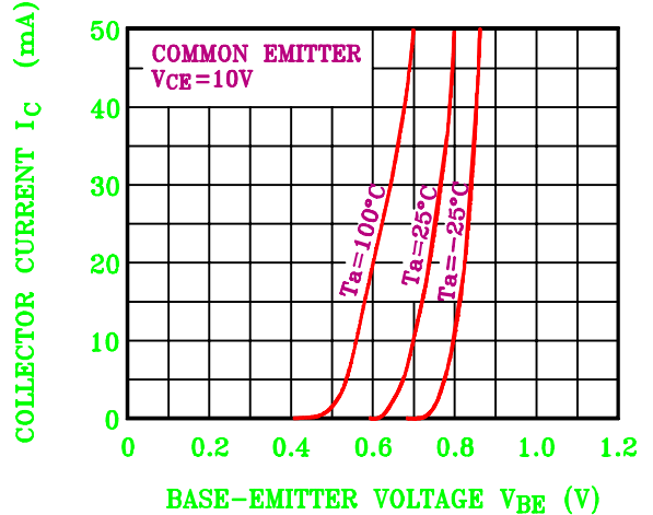
I_C - V_{BE}
