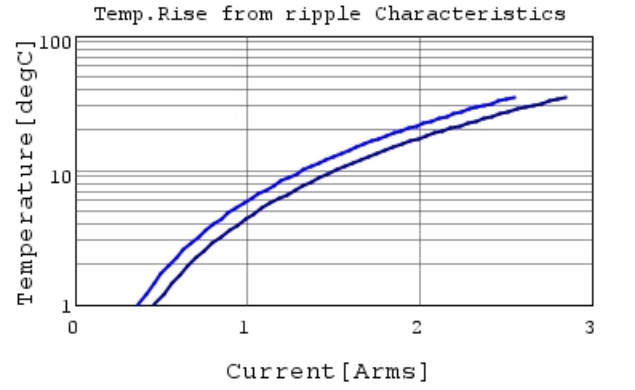
GCM155C71A105KE38 Temp.rise — 500kHz
