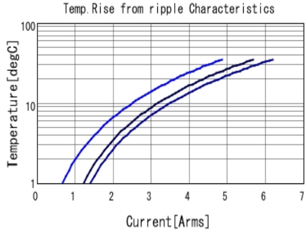
GRM32ER71E226ME15 Temp. rise ■ 80kHz ■ 400kHz ■ 800kHz
