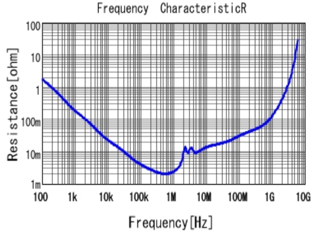
■ GRM32ER71E226ME15 R DCOV, 25degC
