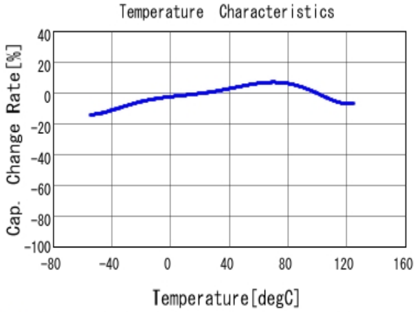
■ GRM32ER71E226ME15 C-Temp. capchange, DCO. 0V, ACO. 5V rm
