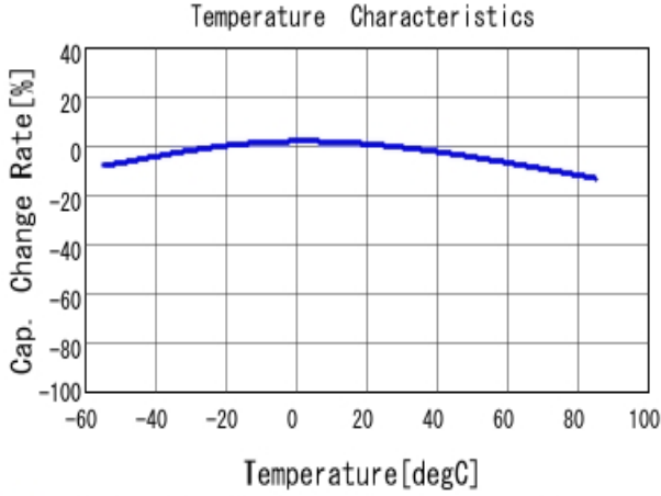
■ GRT155R61E225KE13 C-Temp. capchange, DCO. 0V, ACO. 2V rm
