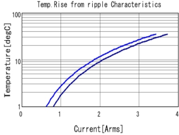
■ GRT155R61E225KE13 Temp. rise ■ 500kHz ■ 1MHz
