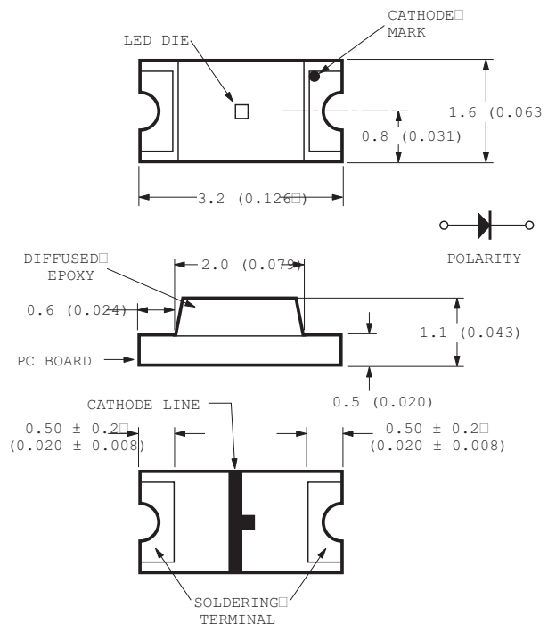
HSMB-C150
