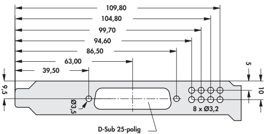
D-Sub 25-polig
