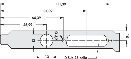
D-Sub 25-polig
