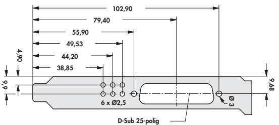
D-Sub 25-polig
