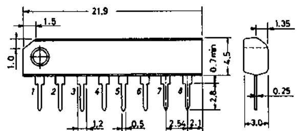
外形図 (単位: mm)
