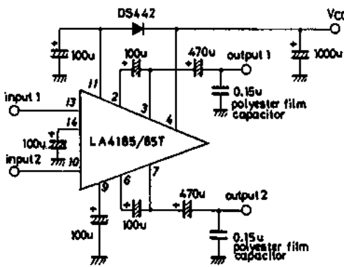
対策回路例
