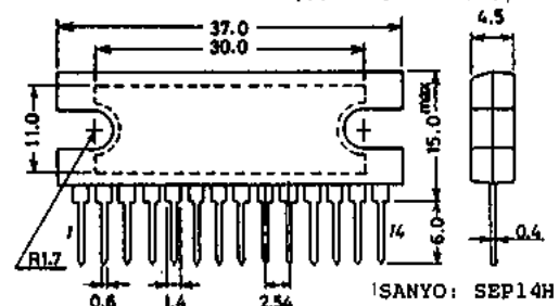
外形図 3023A-S14HIC (unit: mm)
