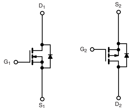
P-Channel MOSFET
