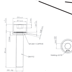
M4 - G2 M4 20x1 CAPSIVE DN-F12 Marking A2-70 A2-70
